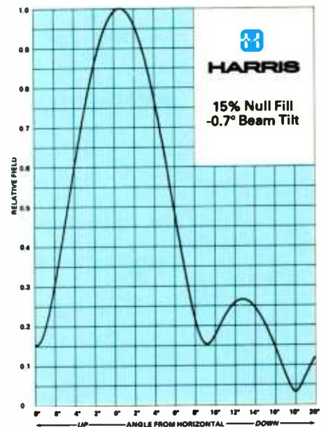
TAB-6H
