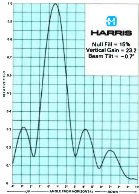
TAZ-24U 3-bay
