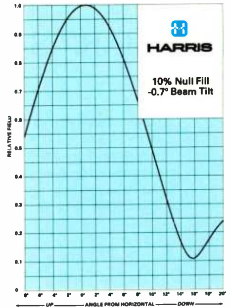
TAB-4L
