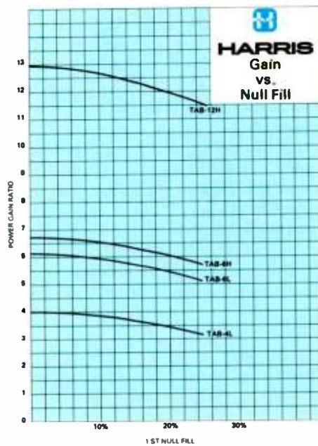
TAB-12H
